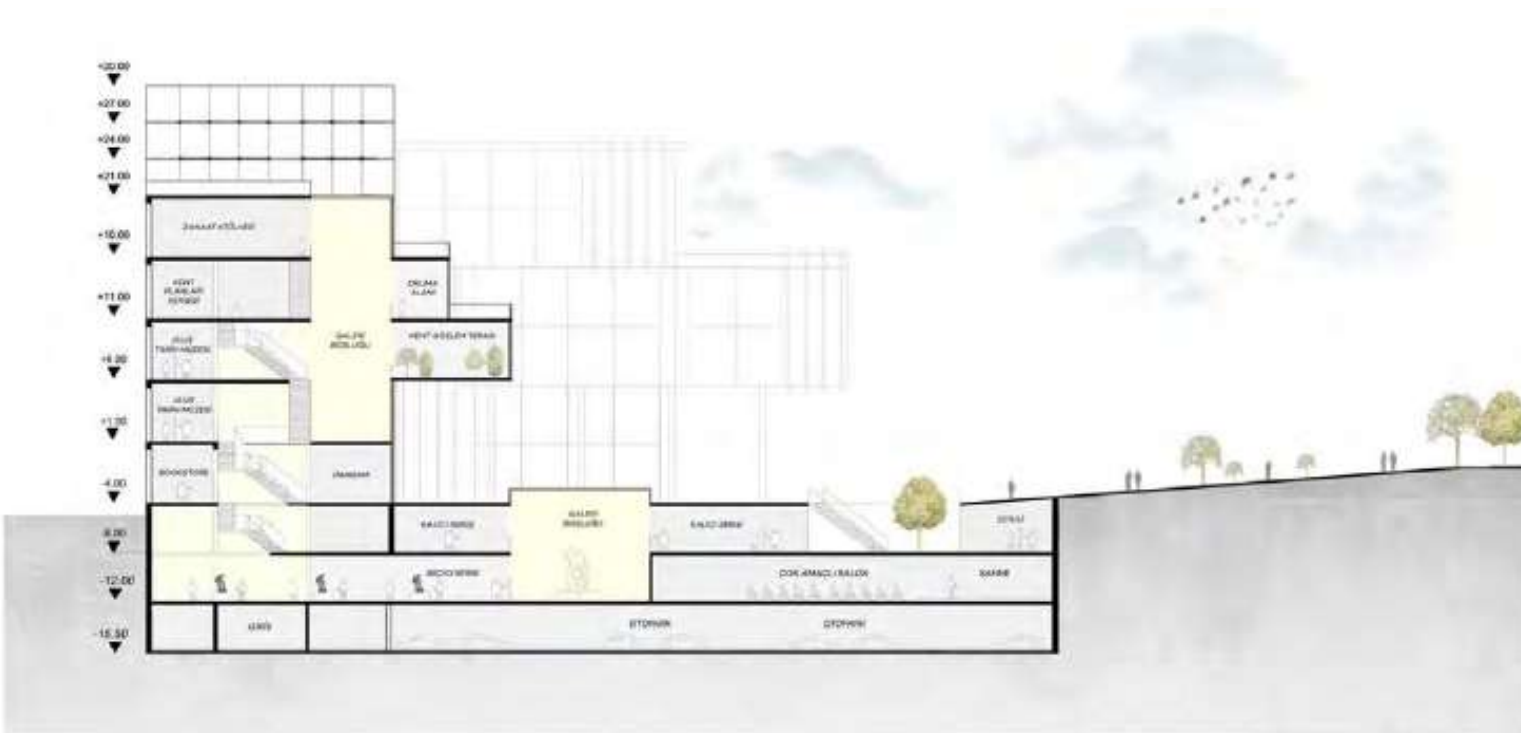
B-B KESİT 1/200
