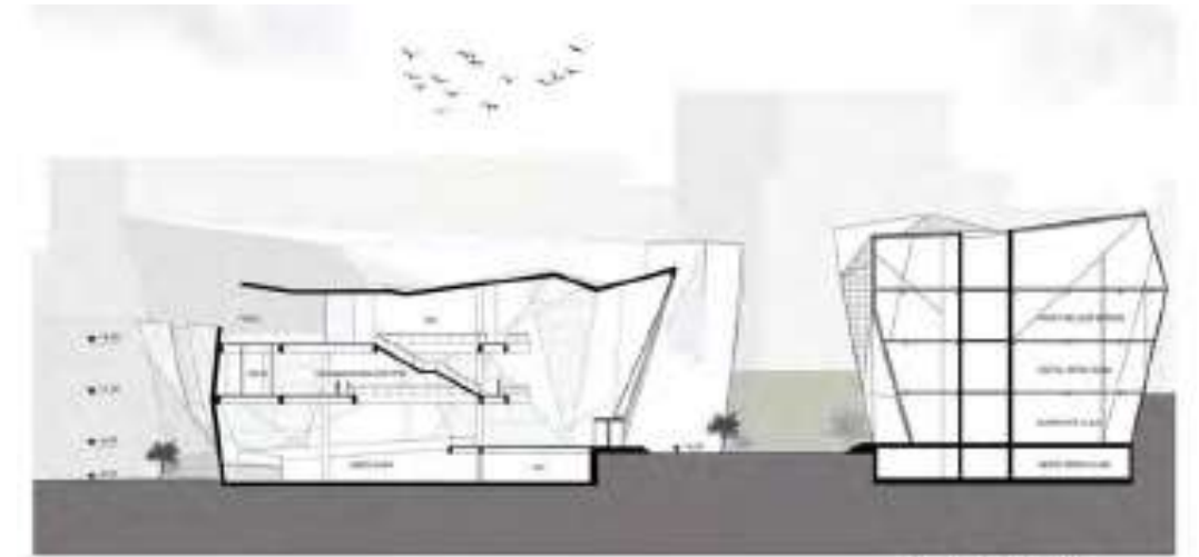
AA KESİT 1/200
